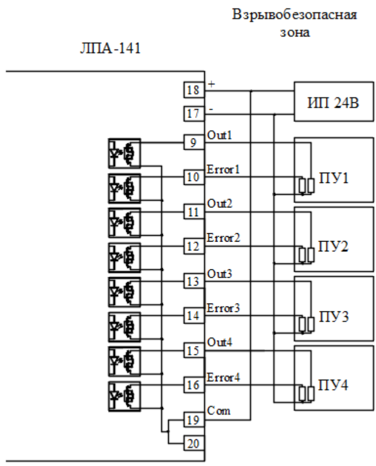
Рисунок 15. Схема подключения барьера ЛПА-141-401 к приемным устройствам, объединенным отрицательным общим проводом
