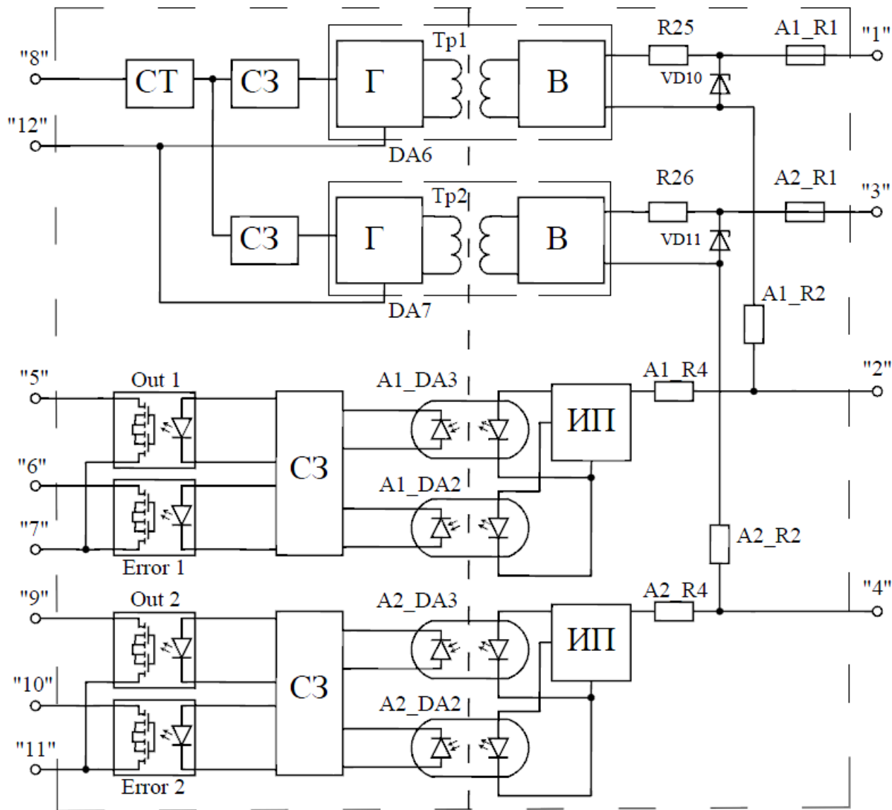
Рисунок Б.1 Структурная схема барьера ЛПА-140-201
