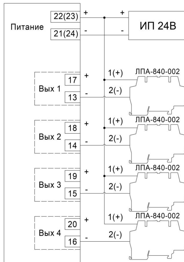
Рисунок 10. Схема подключения к выходу ЛПА-131 релейных модулей ЛПА-840-002 с общим плюсом
