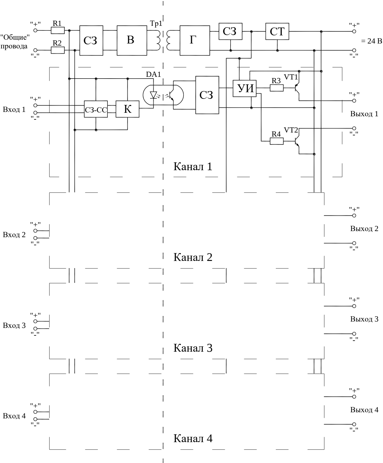
Рисунок Б.1 — Структурная схема барьера ЛПА-131-4XX
