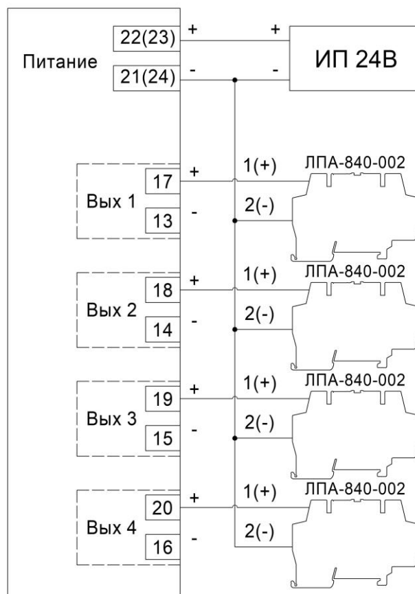
Рисунок 9. Схема подключения к выходу ЛПА-131 релейных модулей ЛПА-840-002 с общим минусом
