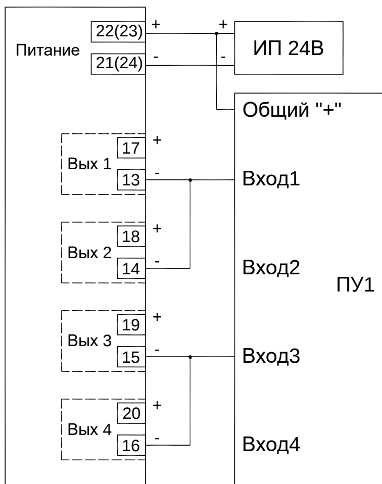
Рисунок 8. Схема подключения выходных цепей барьера ЛПА-131 по схеме «логическое ИЛИ»
