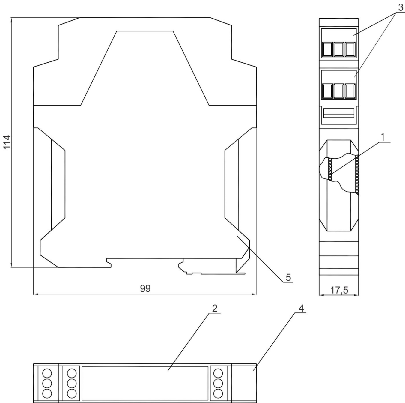
Рис.А1. Конструкция барьера БИА-101
