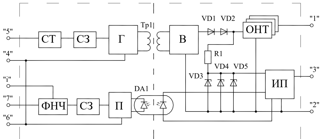
Рис.Б1. Структурная схема барьера БИА-101
