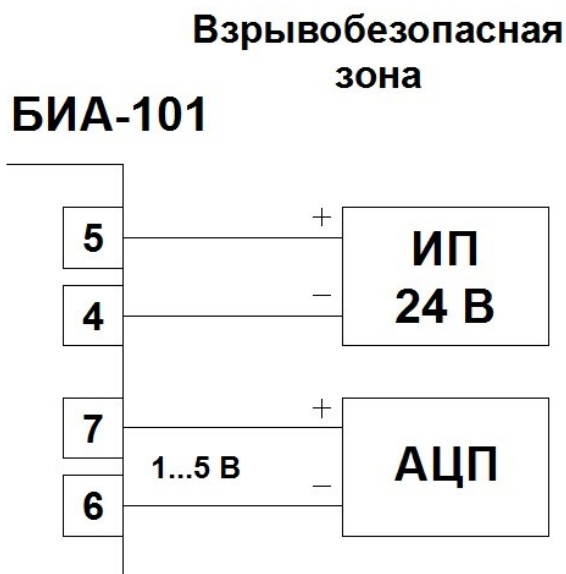
Рис.6. Подключение к потенциальному выходу барьера БИА-101.
