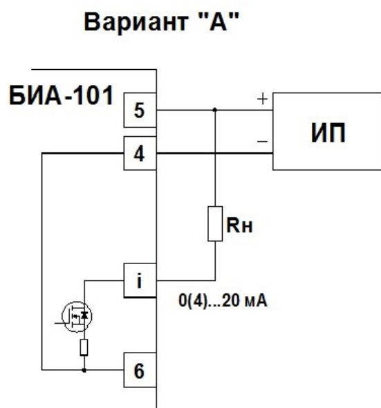
Рис.7. Подключение к токовому выходу барьера БИА-101. Вариант «А» - с общим источником питания, вариант «Б» - с отдельными источниками питания.
