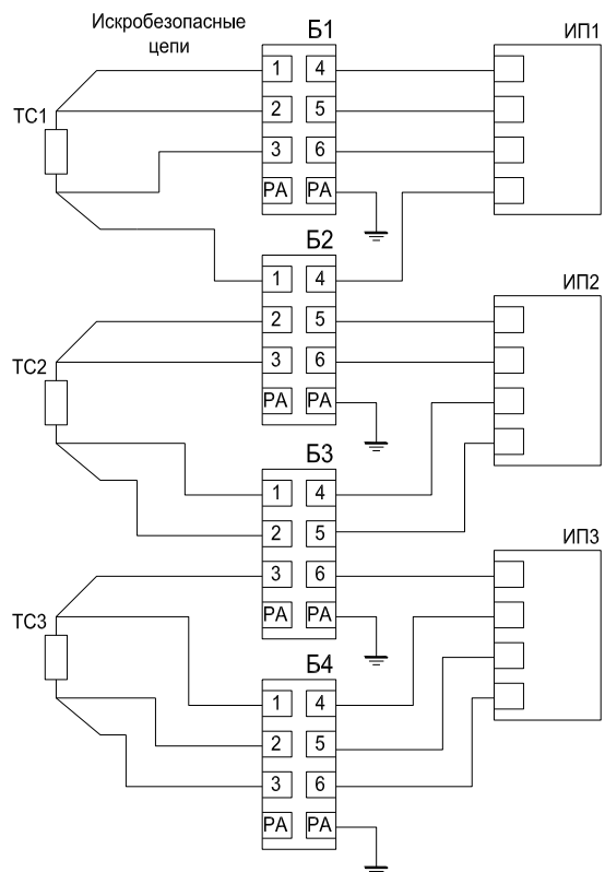
Рис. 3. Четырехпроводная схема подключения термопреобразователя сопротивления (ТС)
